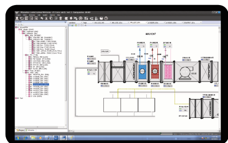
流程图组态
