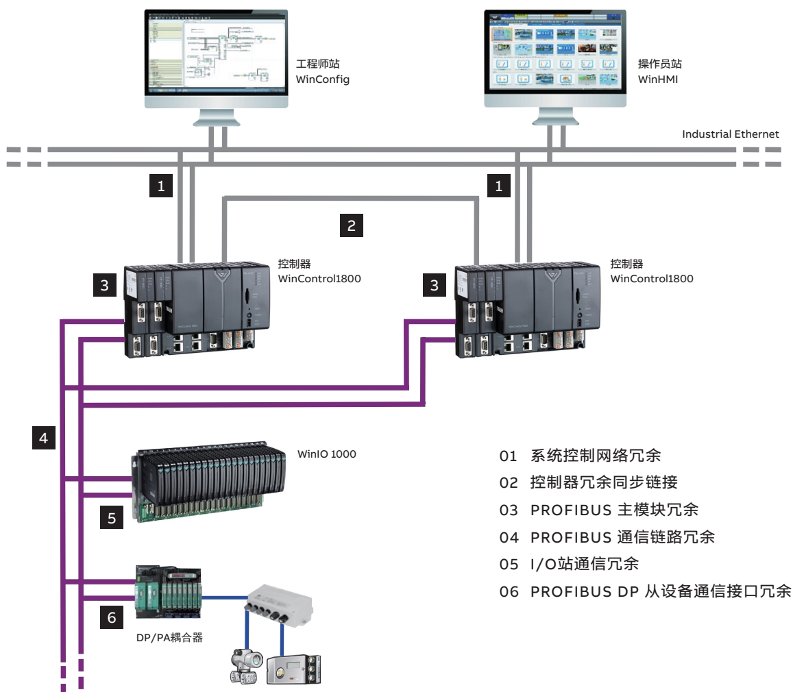
冗余配置图
