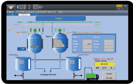
流程图显示
