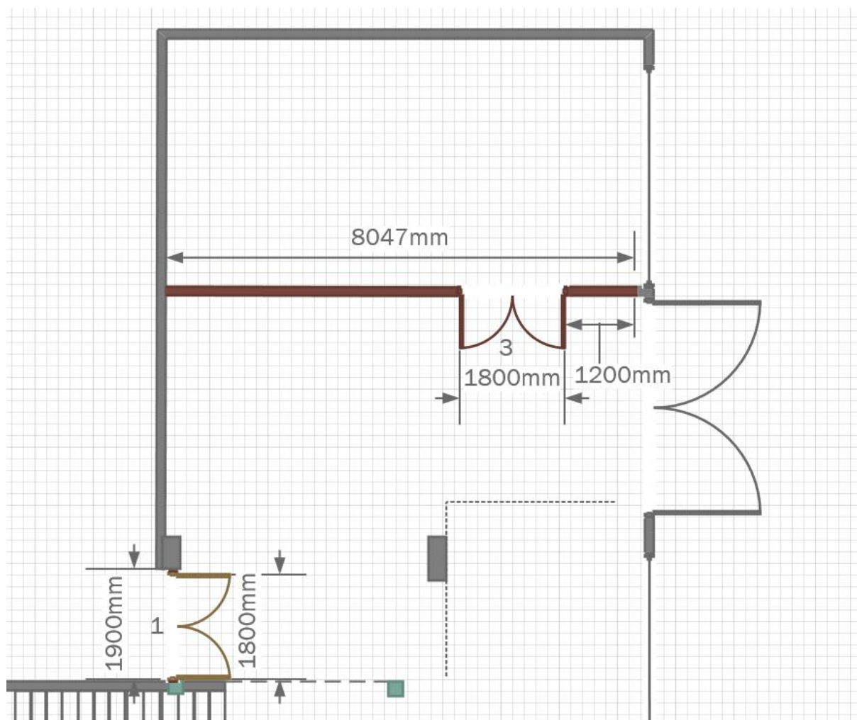
Rys.1. Rozmieszczenie drzwi do chronionych stref oraz wymiary ogrodzeń.
