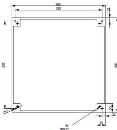
Boorpatroon
