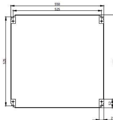
Montageplaat
